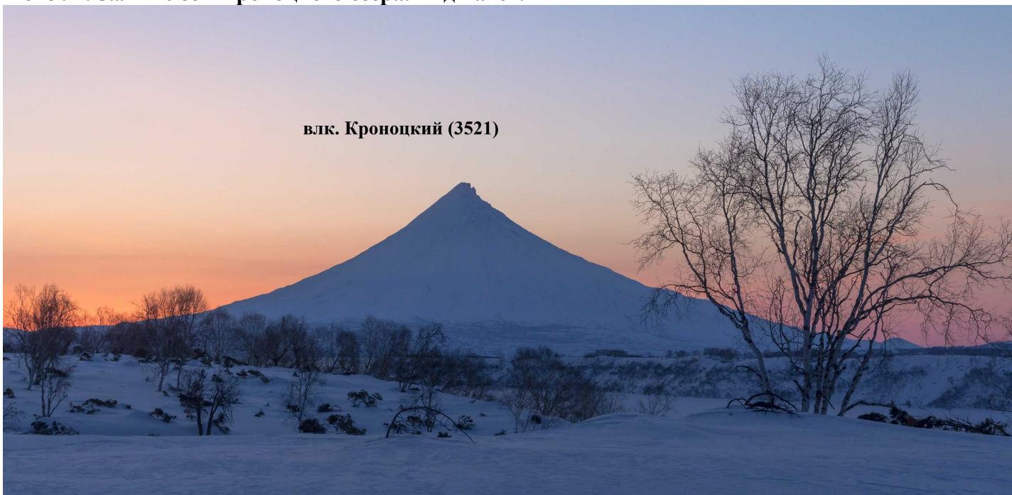
Фото 93. Кроноцкий вулкан
