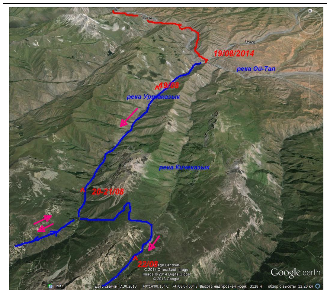
Рисунок 1 Карта К-42-125 (1 км.)
